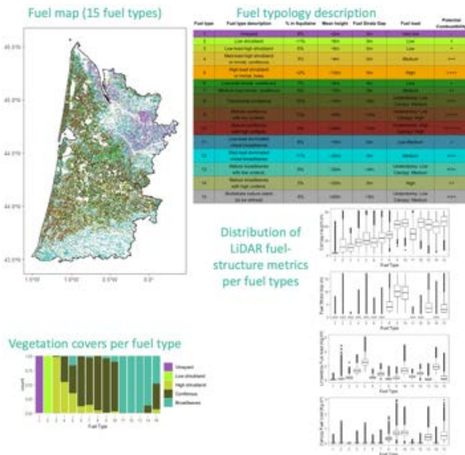
Figure 5.1. Cartographie du combustible dans le massif landais (Gironde et Landes) issue de la combinaison de trois produits de télédétection (LiDAR HD, Cosia et OCS-GE). Cette carte produite à 20 m de résolution permet de cartographier quinze grands types de structures combustibles et de connaître précisément localement le type de couvert ou des valeurs de
