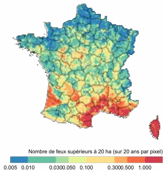
Figure 1.1. Projections du nombre de feux supérieurs à 20 ha selon la TRAAC (maille SAFRAN 8 km)
