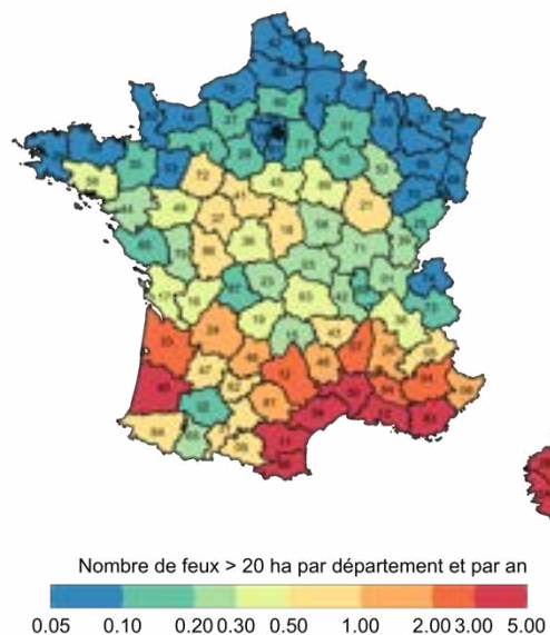
Figure 1.2. Projections du nombre de feux supérieurs à 20ha selon la TRAAC (par départements)
